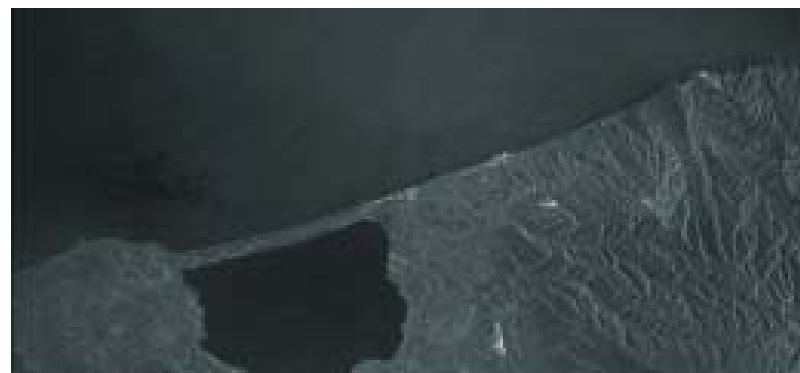
Immagine COSMO-SkyMed del lago di Varano. © 2007 ASI
