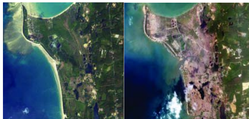
Costa della Thailandia prima e dopo lo tsunami. © Ikonos/Spaceimaging
